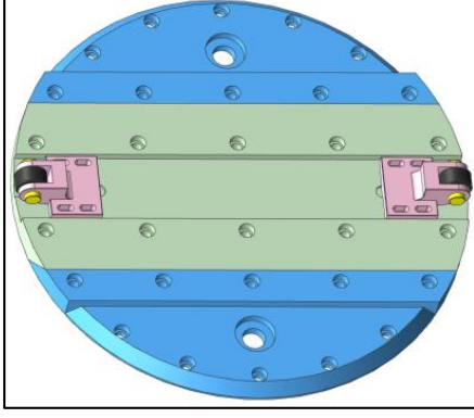
Fig. 4 York & Roller
